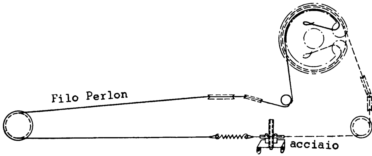
FUNICELLA DELLA MANOPOLA SINTONIA FM
