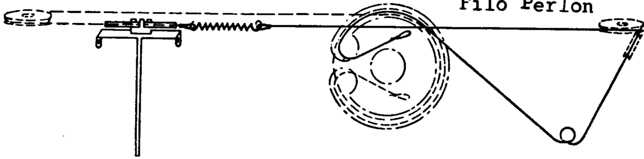
FUNICELLA DELLA MANOPOLA SINTONIA AM
